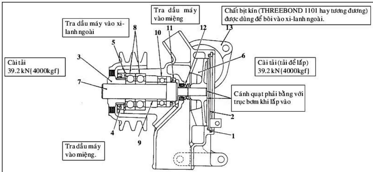
Hình 4.23. Kiểm tra các chi tiết sau khi lắp
