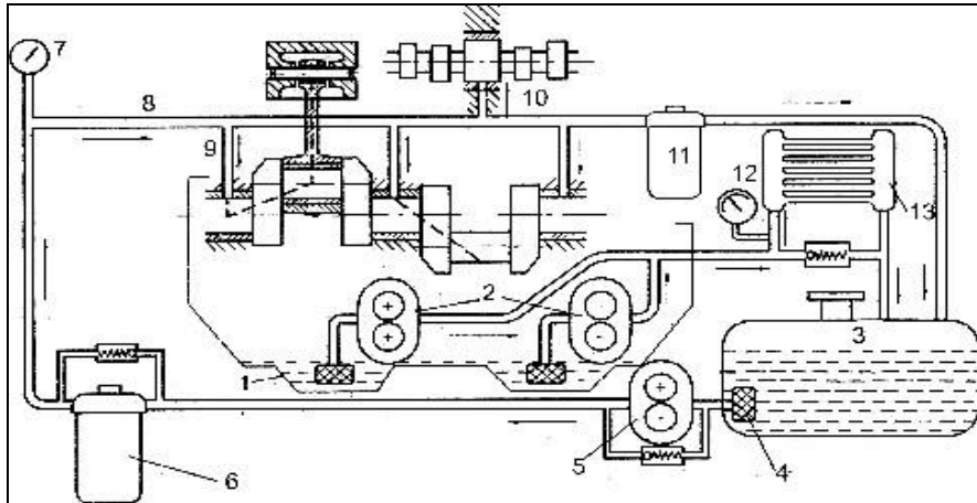
Hình 1.5. Hệ thống bôi trơn các te khô
