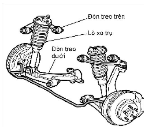
Hình 1.35. Hệ thống treo độc lập
