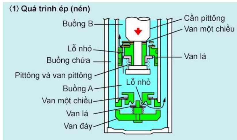
Hình 1.30. Hành trình ép bộ giảm chấn kiểu kép +Tốc độ chuyển động của cần pittông cao:
