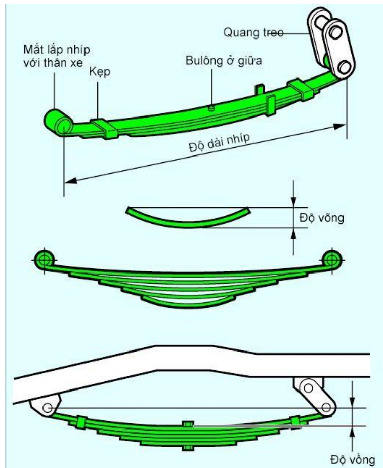
Hình 1.18. Nhíp lá * Đặc
