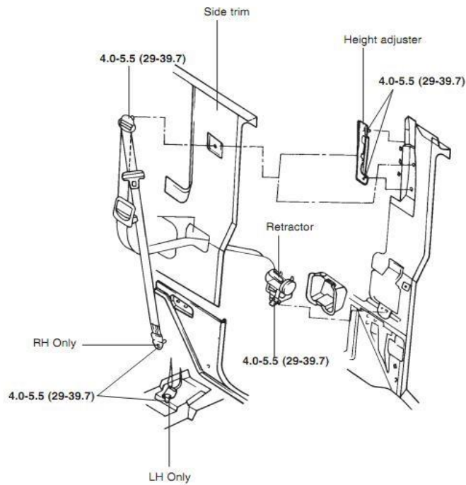
Hình 4.7. Đai an toàn cho người lái
