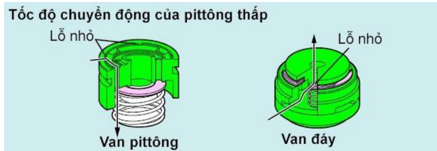
Hình 1.33. Hành trình hồi vị khi piston ở tốc độ thấp 1.3.3 Bộ phận dẫn hướng
