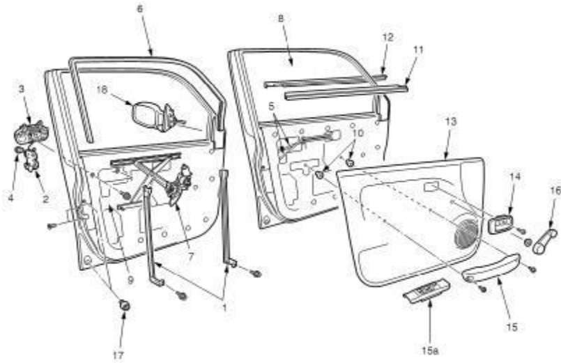
Hình 4.11. Các chi tiết cửa xe con
