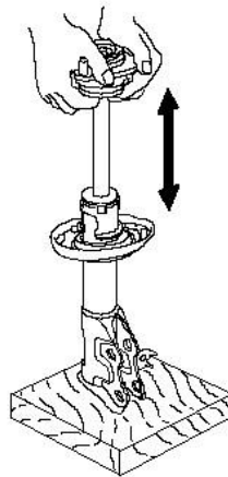
Hình 3.5. Kiểm tra giảm sóc
