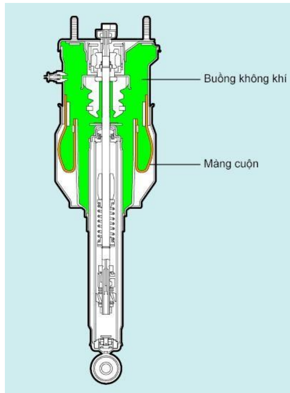
Hình 1.23. Lò xo không khí
