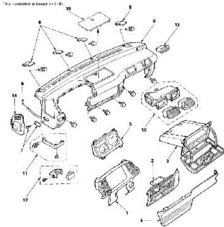
Hình 4.9. Các chi tiết trong cabin xe
