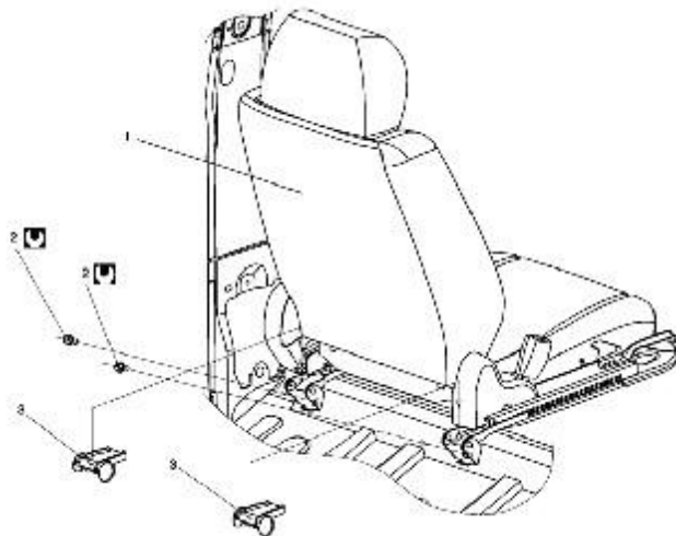
Hình 4.6. Ghế đệm lắp trên xe
