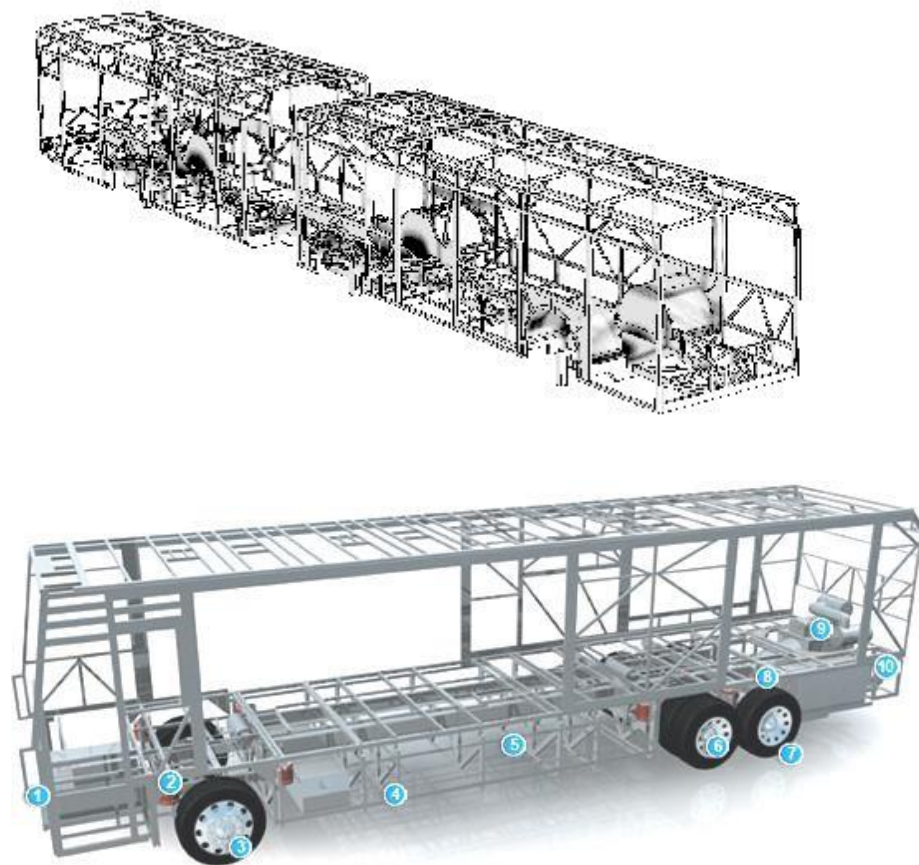
Hình 4.3. Khung xe chở khách
