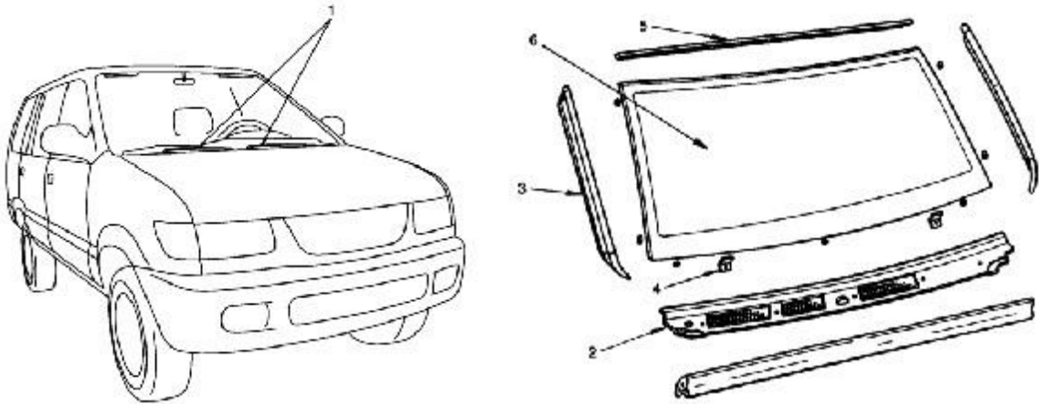
Hình 4.12. Kính chắn gió phía trước
