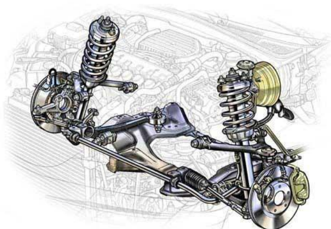
Hình 1.11. Hệ thống treo trên xe Panamera
