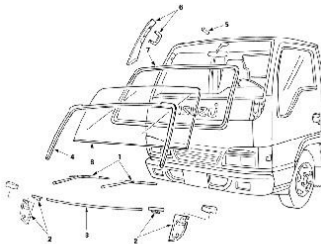
Hình 4.10. Kính chắn gió lắp trên xe
