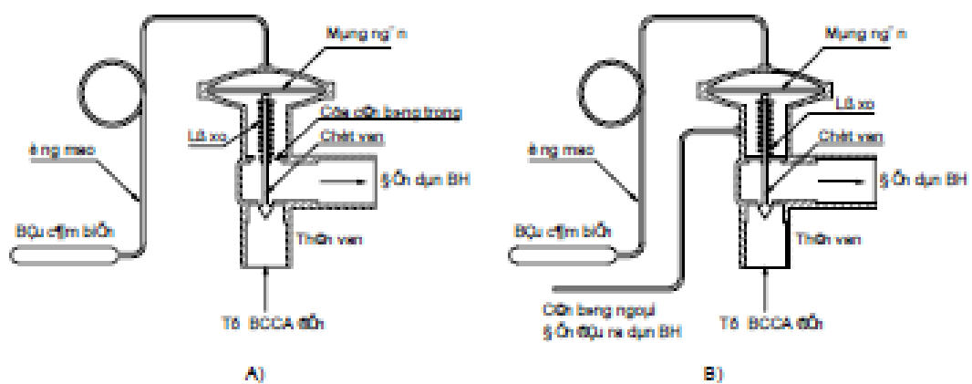
Van tiết lưu tự động
