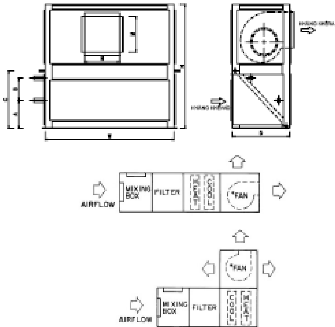
Cấu tạo bên trong của AHU
